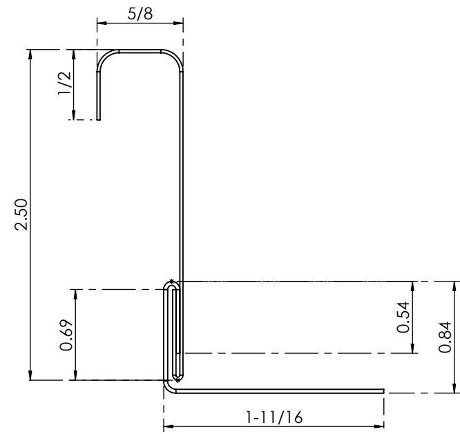
ELEVACION ESC. 1:1
