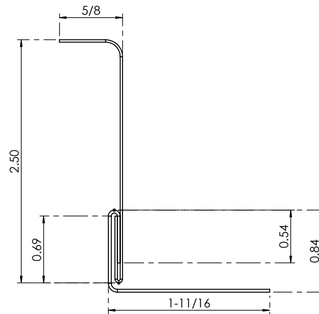
ELEVACION ESC. 1:1
