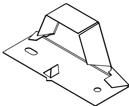
ISOMETRICO
