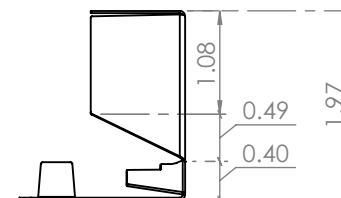
VISTA LATERAL
