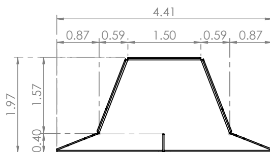
ELEVACION
