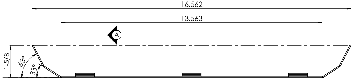
ELEVACION
