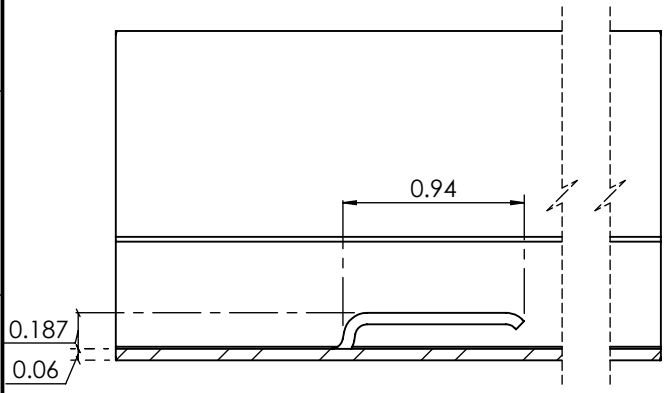
SECCION "A-A" ESC. 1:1
