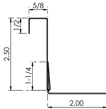
ELEVACION
