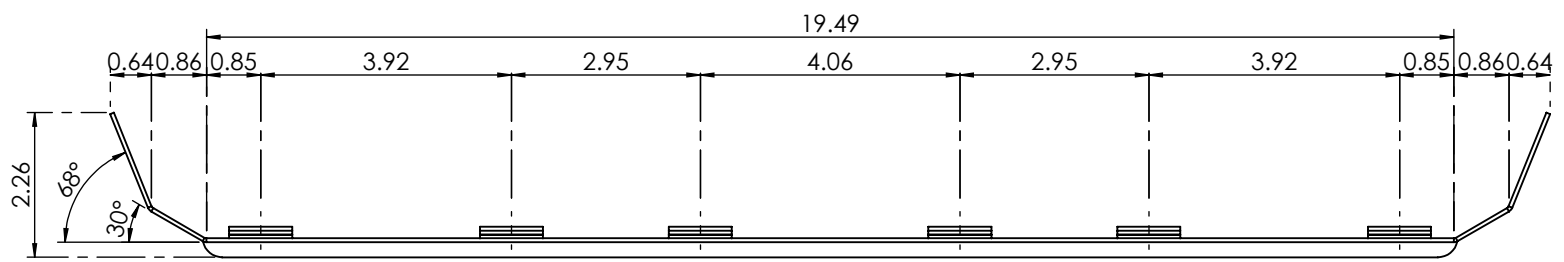
ELEVACION
