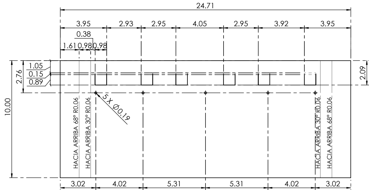
VISTA DESPLEGADA
