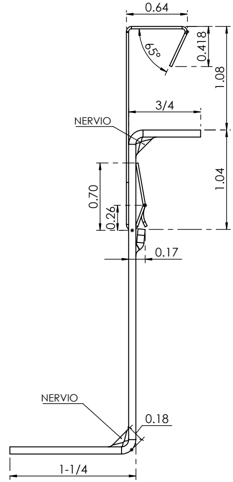
VISTA LATERAL ESC. 1:1
