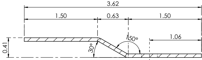
SECCION ELEVACION ESC. 1:1
