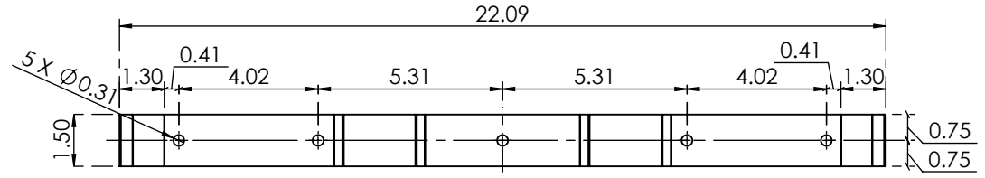
PLANTA ESC. 1:5
