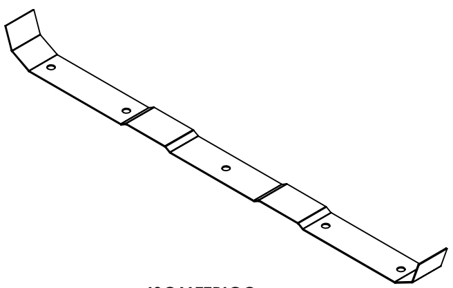
ISOMETRICO
