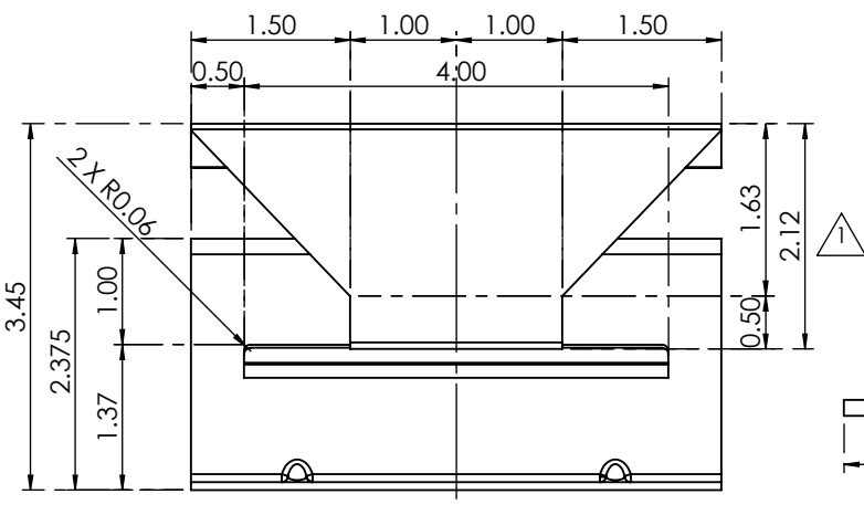
ELEVACION
